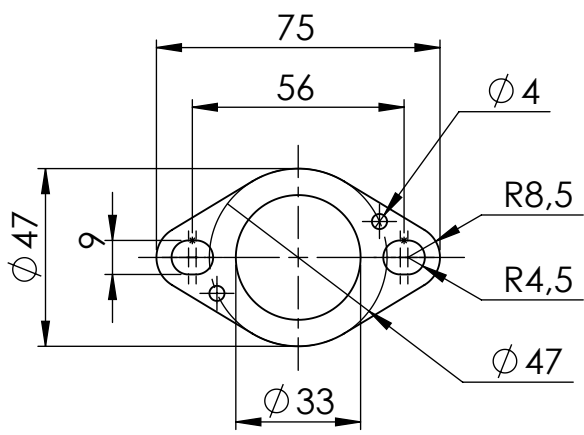
Flange 45E Cod.205267
