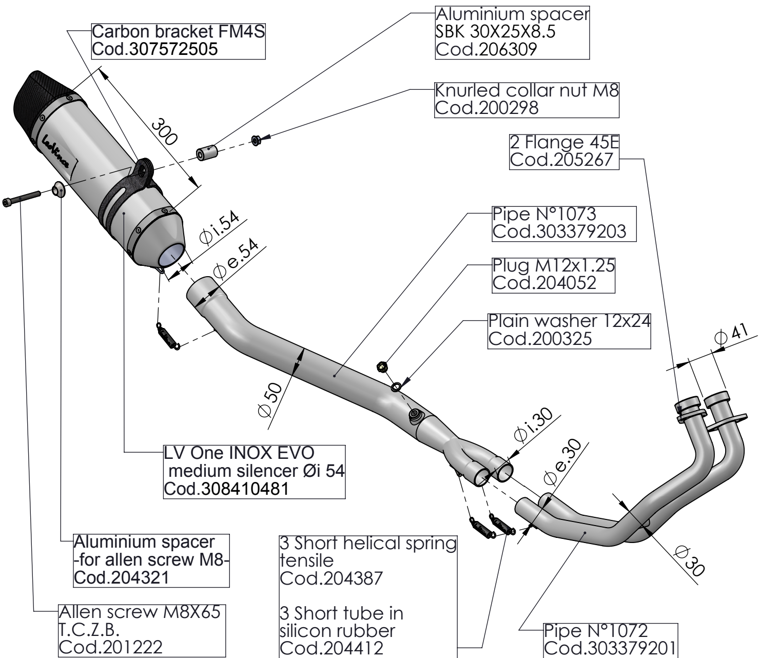
Flange 45E Cod.205267
